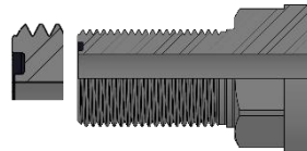
SAE J1453 / ISO 8434-3 (ORFS Pasatabique)
